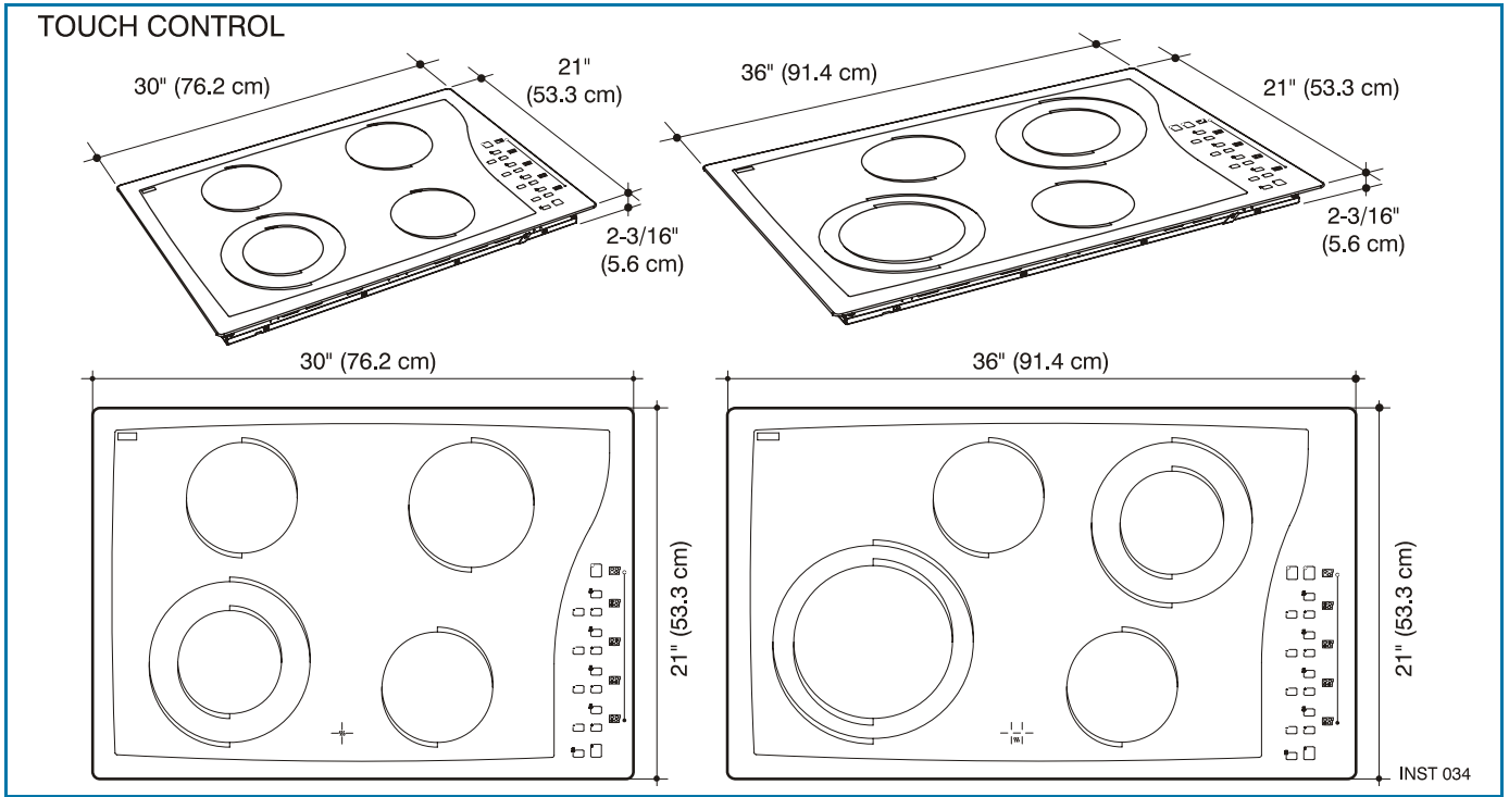
Figura 1. Touch control electrónico
